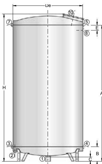
PASSO D'UOMO DECENTRATO PER MODELLI DA 3000 A 15000
